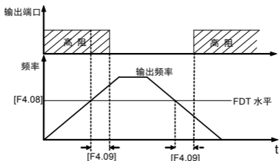
图 6-14 频率水平检测信号 (FDT)
