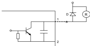
图 6-12 OC 输出端子的内部线路
