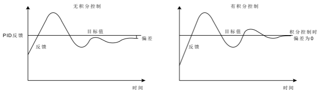
图 6-18 积分控制的作用
